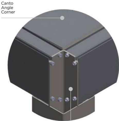
Detalhe interior sem coluna/poste Détail intérieur sans colonne/poteau Interior detail without column/post
