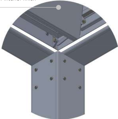
Acabamento interior do canto Finition intérieure d'angle Corner interior finish
